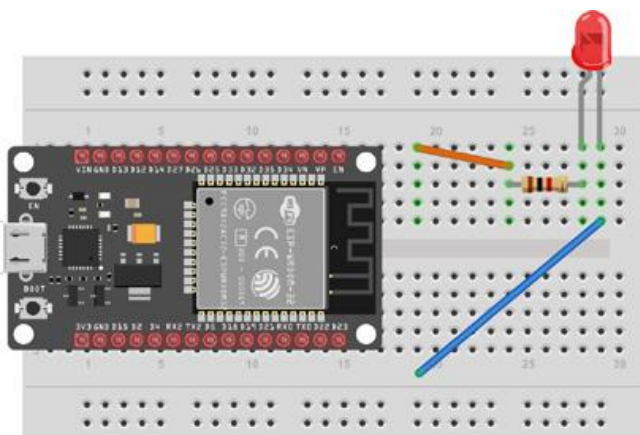
Abb. 1.4: ESP32 auf Steckbrett – fehlende Pins für Anschluss
