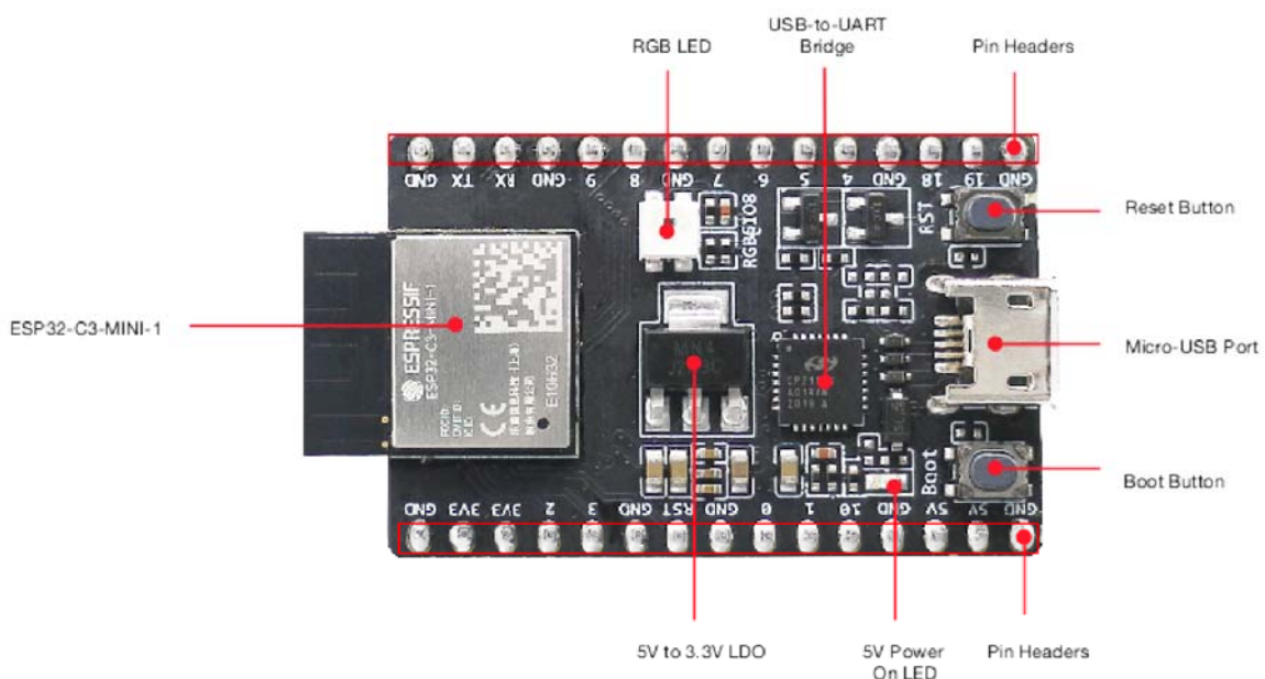
Abb. 2.2: ESP32-C3-DevKitM-1 (Quelle: Espressif)
