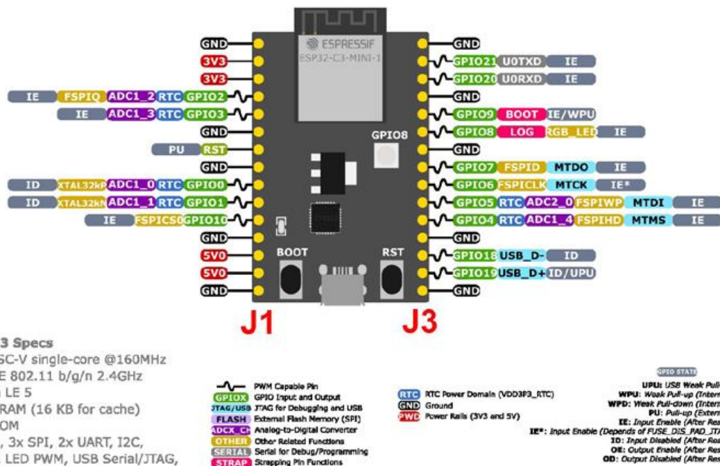
Abb. 2.3: ESP32-C3-DevKitM-1 – Anschlussbelegung (Quelle Espressif).
