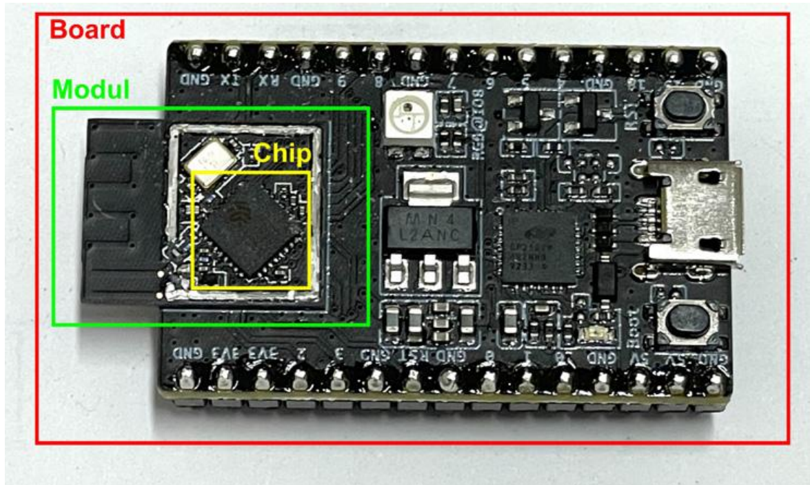
Abb. 2.1: ESP32-Kategorien – Board (rot), Modul (grün), Chip (gelb)
