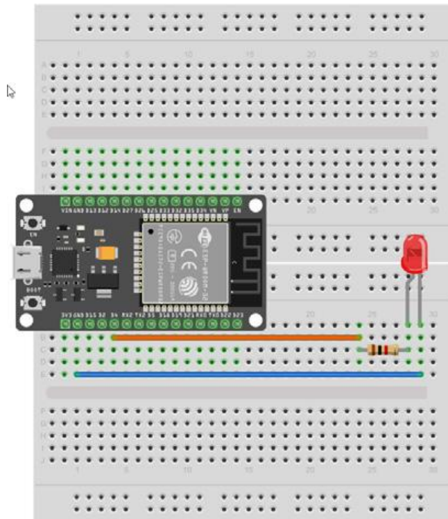
Abb. 1.5: ESP32 auf Steckbrett (Variante mit zwei Boards)
