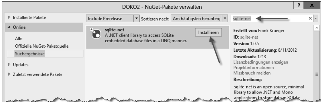
Abbildung 10.16 NuGet-Paket installieren
