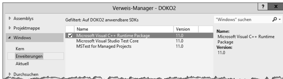
Abbildung 10.14 Verweis hinzufügen
