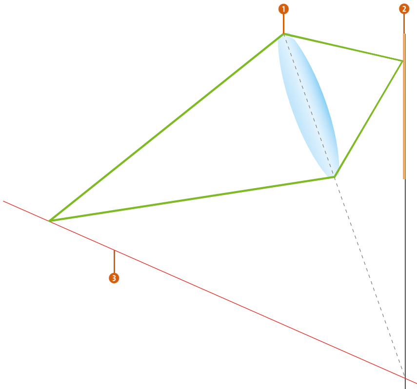
▲ Abbildung 3.41 Wenn Sensorebene (orange 2) und Objektiv (blau 1) nicht mehr parallel zueinander stehen, kippen Sie damit die Schärfeebene (rot 3) im Raum. Sensorebene, Objektivenebene und Schärfeebene schneiden sich dabei nach der Scheimpflug'schen Regel in einer Geraden.
