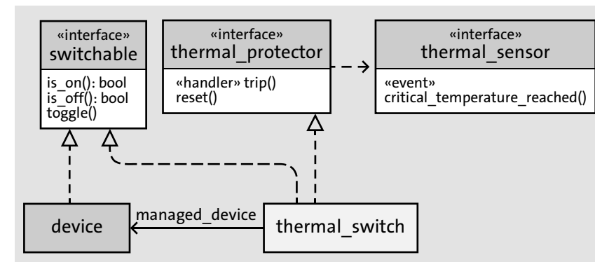
Abbildung 4.1 Die Klasse thermal_switch und das Interface thermal_protector
