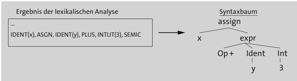
Abbildung 1.4 Ergebnis der Syntaxanalyse (Beispiel)
