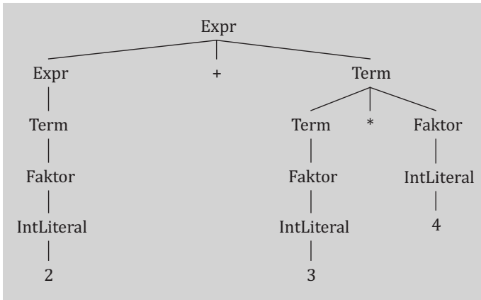
Abbildung 5.3 Syntaxbaum für den Ausdruck »2+3*4«
