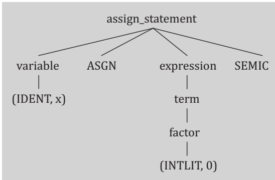
Abbildung 5.6 Teilbaum des Syntaxbaums
