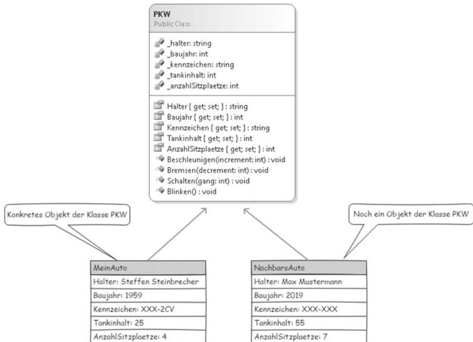
Abbildung 1.9: Konkrete Objekte einer Klasse PKW zur Laufzeit eines Programms.
