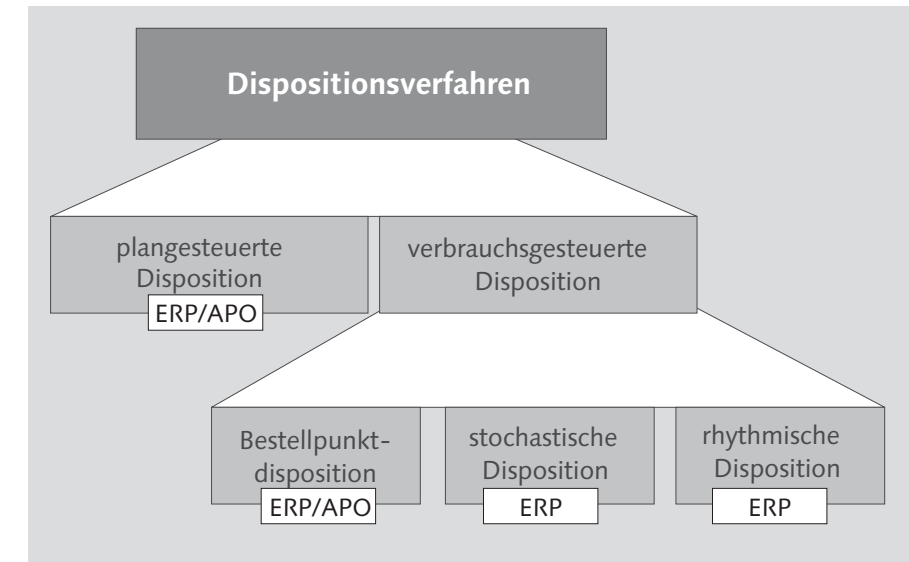
Abbildung 8.12 Dispositionsverfahren im SAP-ERP- und im SAP-APO-System
