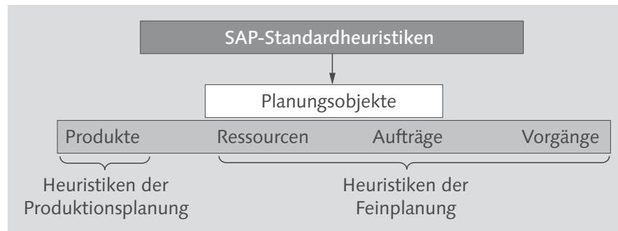
Abbildung 8.9 SAP-Standardheuristiken
