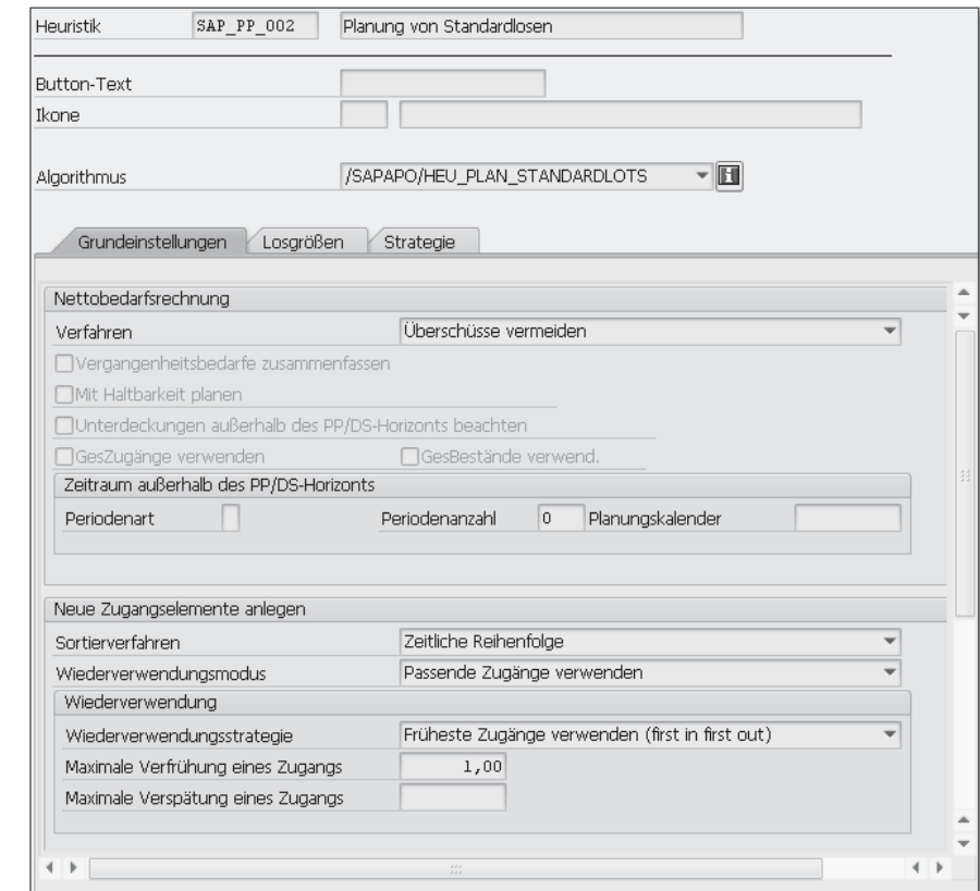
Abbildung 8.8 Auszug der Heuristikeinstellungen der Produktheuristik SAP_PP_002
