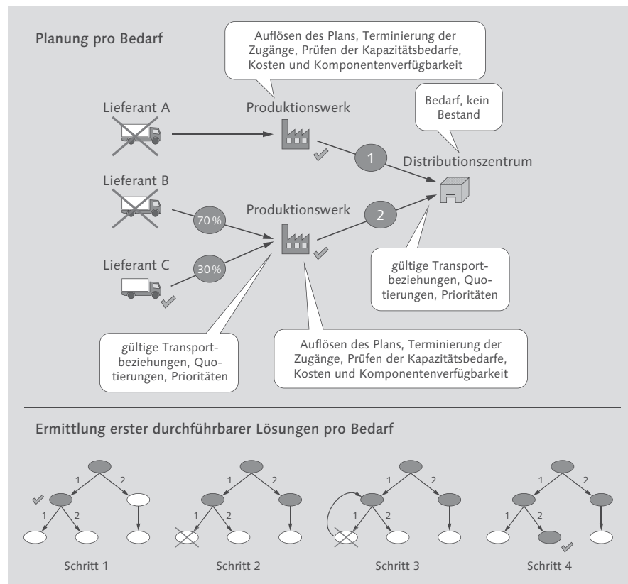
Abbildung 8.15 Planungsszenario CTM (Quelle: SAP)
