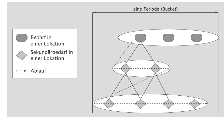
Abbildung 8.14 Verarbeitung SNP-Heuristik (Quelle: SAP)
