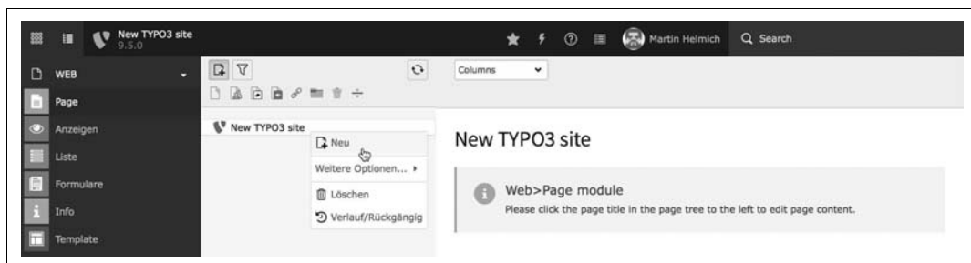
Abbildung 3-8 ▲ Das Pop-up-Menü
